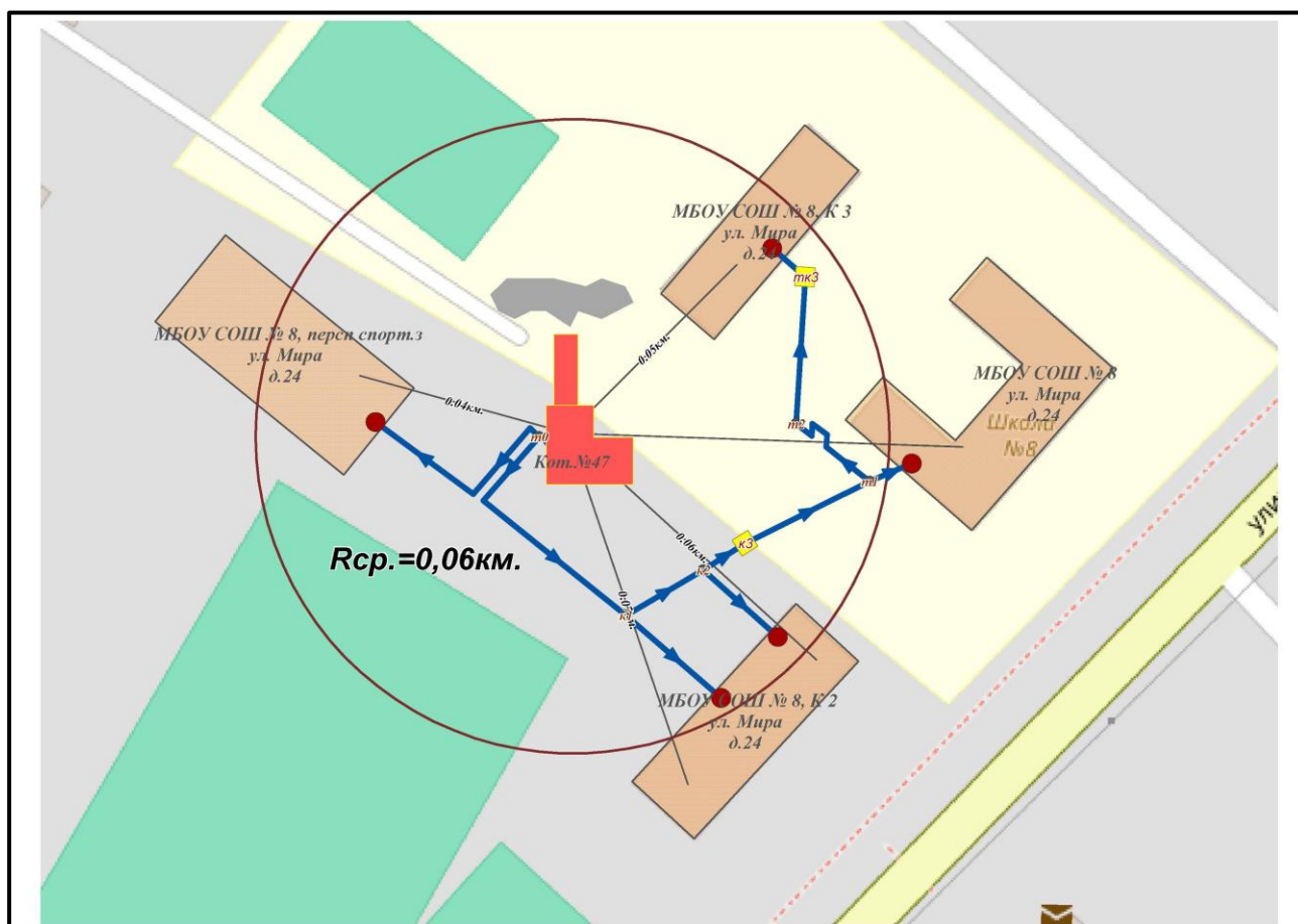
Рисунок 2.5.1 – РЭТС Котельной № 47, п. Сенной
