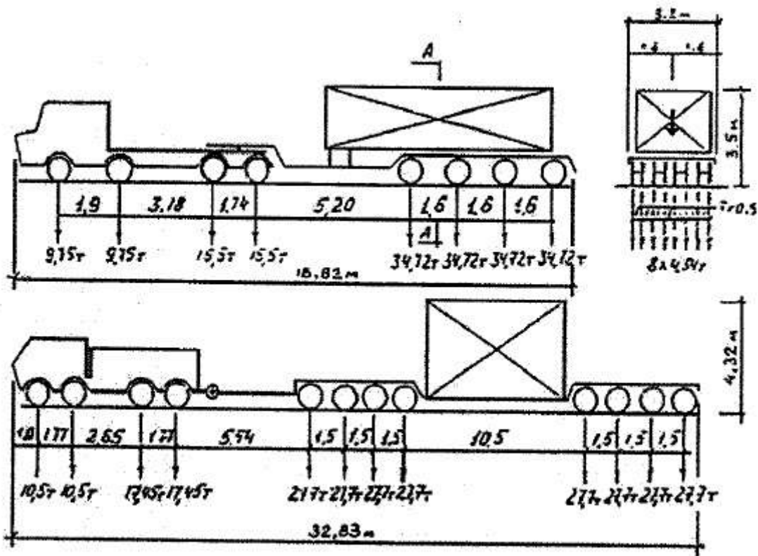
Схема автопоезда
