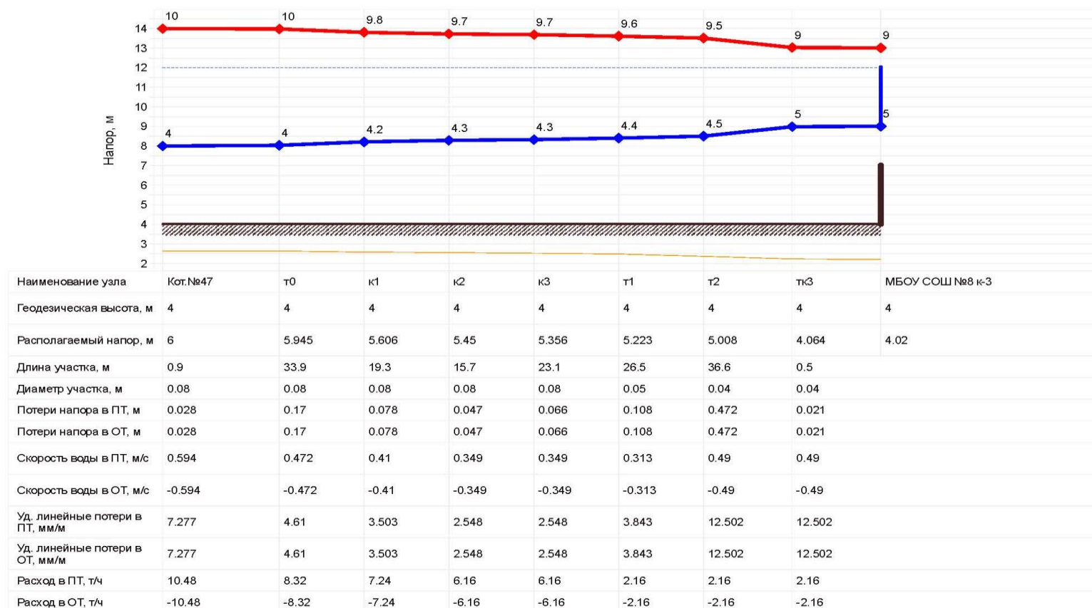
Пьезометрический график от «Кот. №47» до «МБОУ СОШ №8 к-3»
