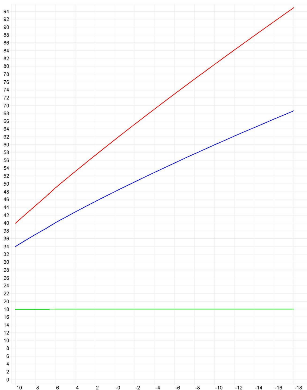
Рисунок 1.3.6.1 – Температурный график Котельных Сенного с. п.
