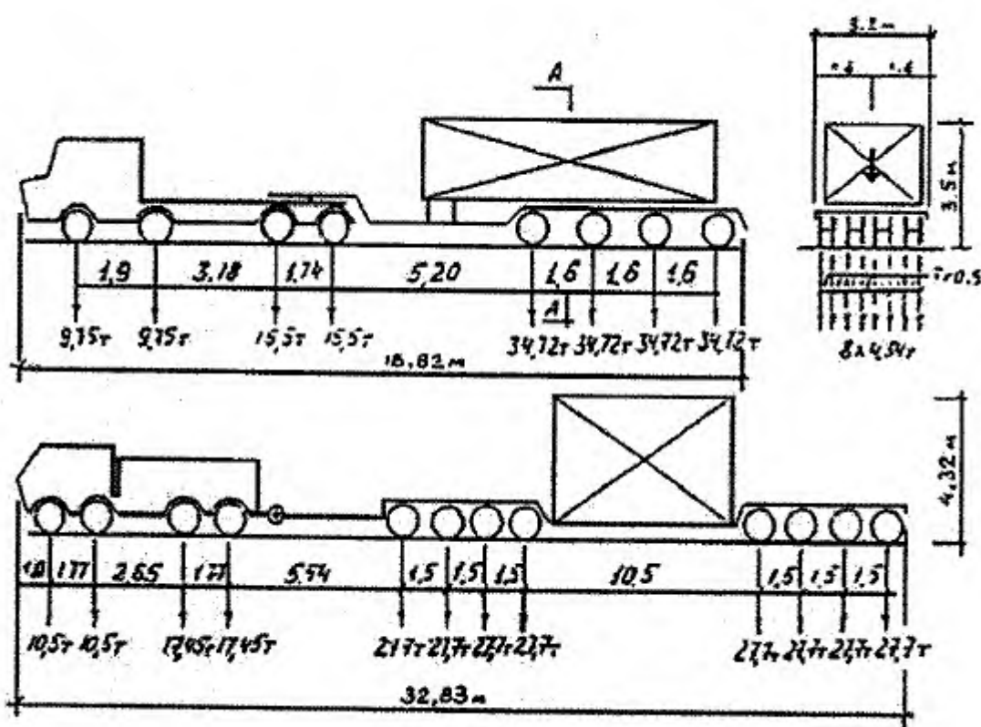
Схема автопоезда
